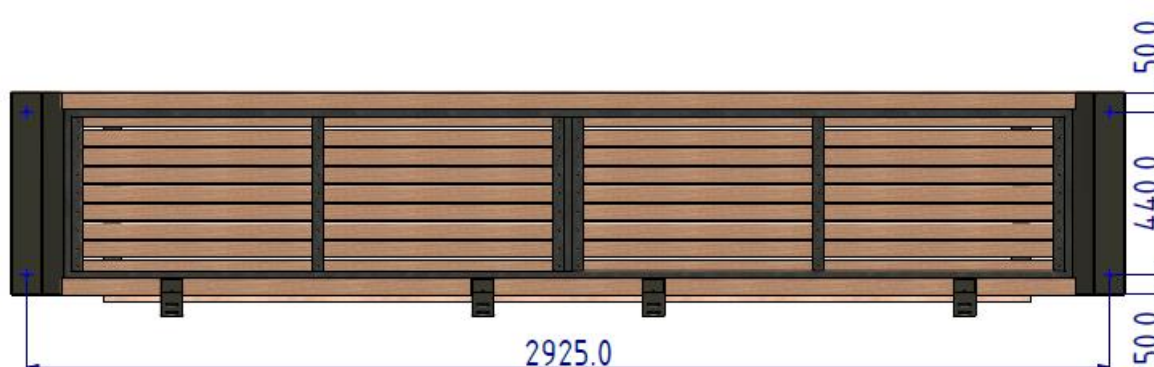
Rzut z wymiarami montażowymi do podłoża.
